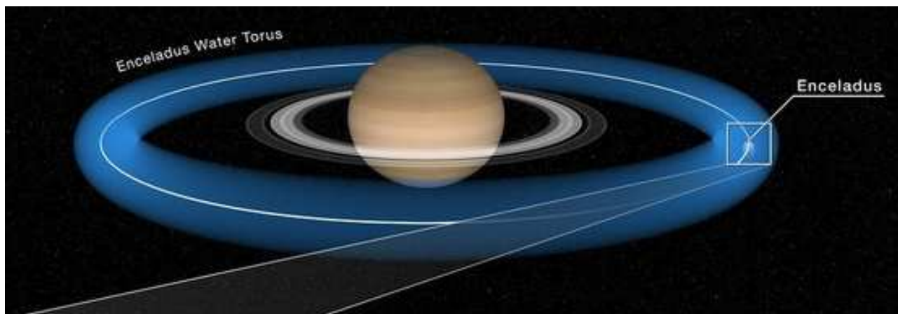
Рис. 3. К определению тора из водяного пара, порожденного Энцеладом вокруг Сатурна.
