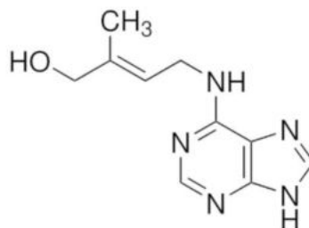
вещество 3
