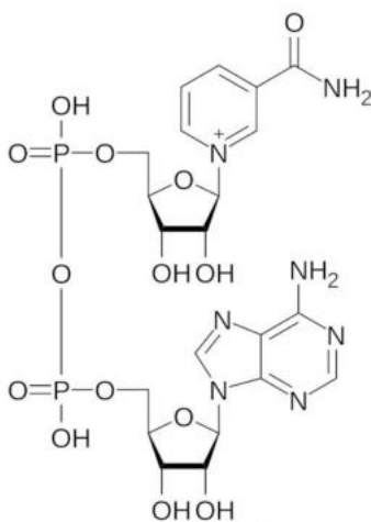
вещество 5
