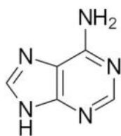
вещество 1
