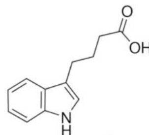
вещество 4
