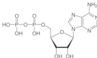
вещество 6
