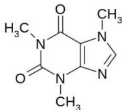
вещество 2
